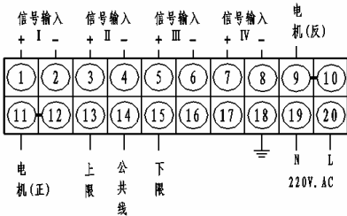
伺服放大器
