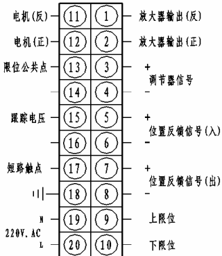
电动操作器
