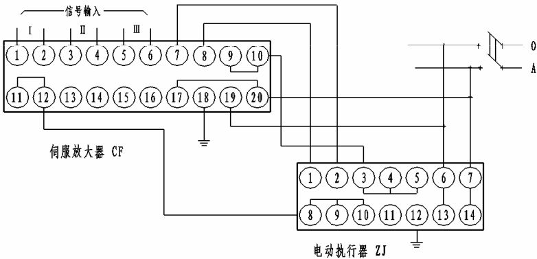
无操作器接线图
